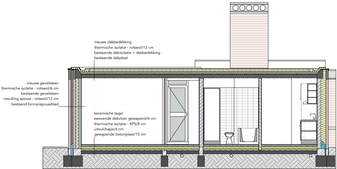
Snede gerenoveerde woning Egelsvennen - beeld: PED architecten
