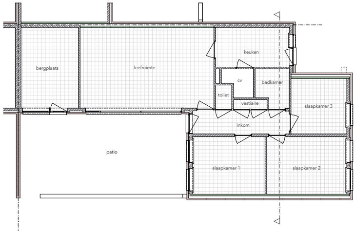
Grondplan bestaande woning Egelsvennen - beeld: PED architecten.
