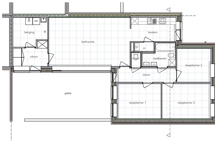
Grondplan gerenoveerde woning Egelsvennen - beeld: PED architecten.
